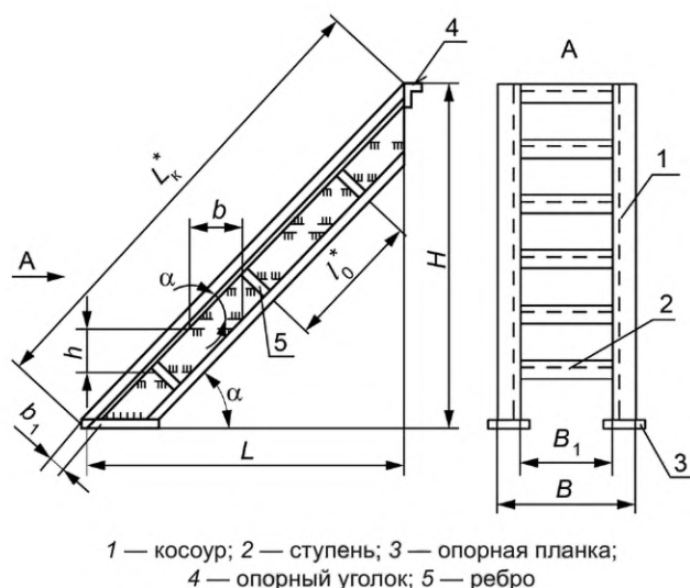
Рисунок 1 — Лестничный марш (МЛ)
