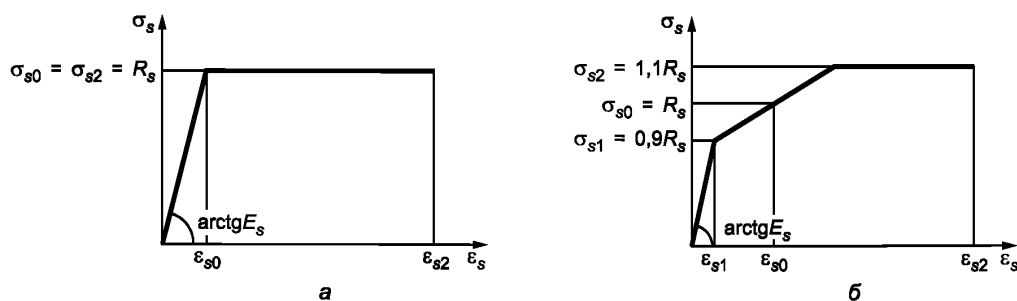
а — двухлинейная диаграмма; б — трехлинейная диаграмма
