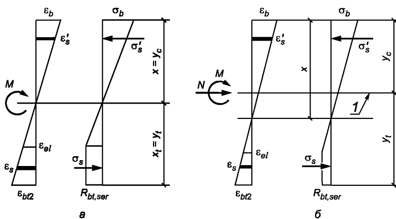
1 — уровень центра тяжести приведенного поперечного сечения
