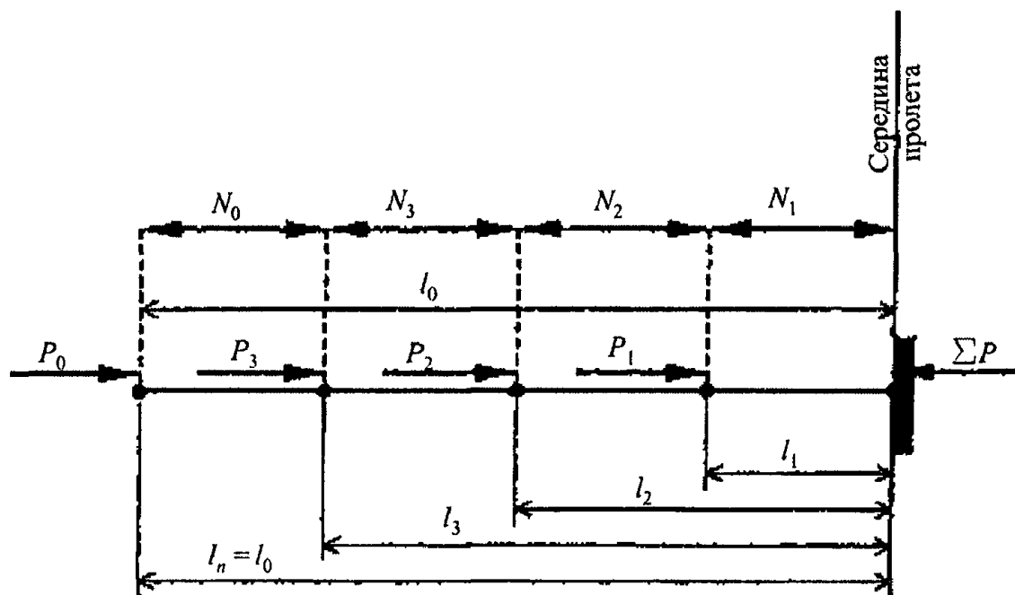
Рисунок К.1 - Расчетная схема сжатых участков пояса фермы
