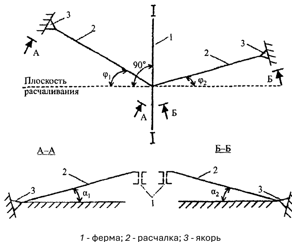
Рисунок К.2 - Схема раскрепления ферм расчалками
